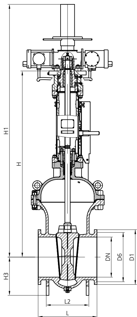
Рис. 1 Фланцевое присоединение
